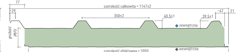
WOOLTECH płyta warstwowa dachowa
