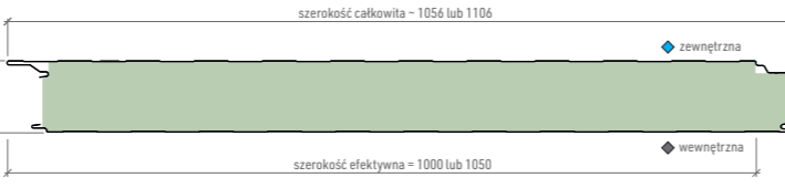
WOOLTECH płyta warstwowa ścienna - plus
