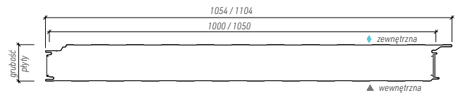
PIRTECH płyta warstwowa ścienna - plus
