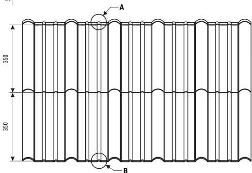
połączenie arkuszy
