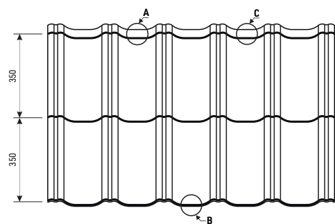
połączenie arkuszy
