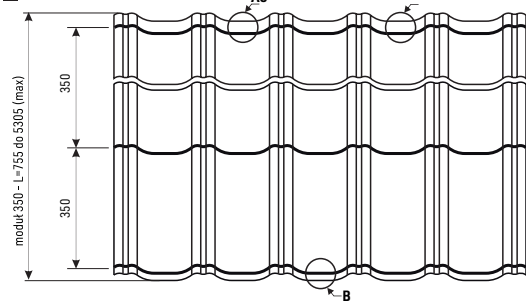
początek arkusza
