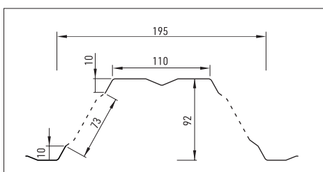
przykład możliwej perforacji T92P
