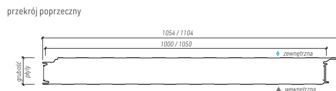
PIRTECH płyta warstwowa ścienna - plus
