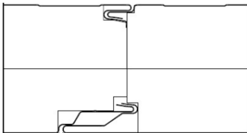
Rys. 1 Płyta ścienna PWS2 – MW - PL – połączenie płyt ze sobą: na „wpust i pióro” (rysunek dostarczony przez zleceniodawcę)
