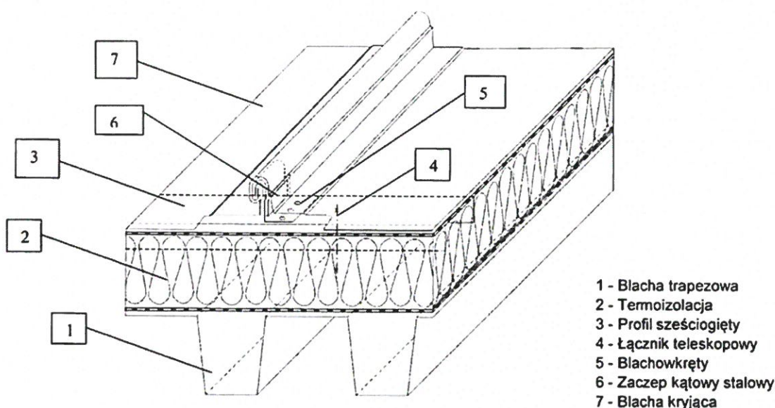
Rys. 1. Schemat dachu systemu DWS TYTANIUM PRUSZYŃSKI (opis w tekście)
