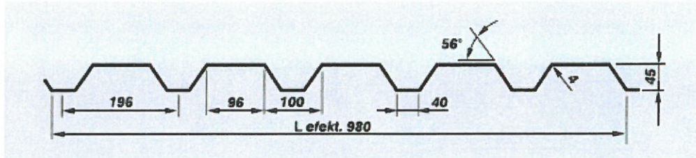
Blacha trapezowa T45 – gr. 0,60; 0,63; 0,70; 0,75; 0,80; 0,88; 0,90; 1,00 mm
