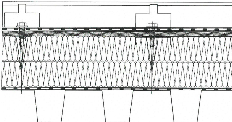
Rys. A3. Przekrój poprzeczny przekrycia dachowego DWW L TYTANIUM PRUSZYŃSKI
