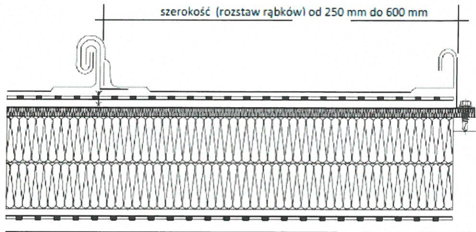
Rys. A2. Przekrój podłużny przekrycia dachowego DWW L TYTANIUM PRUSZYŃSKI
