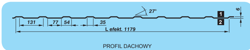
PROFIL DACHOWY
