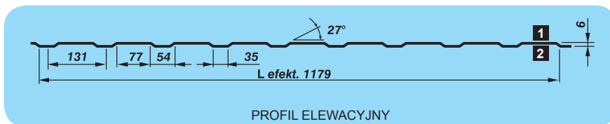
PROFIL ELEWACYJNY
