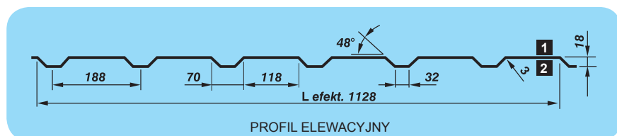
PROFIL ELEWACYJNY
