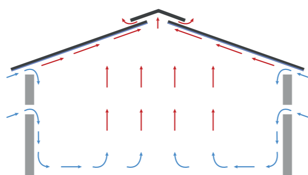
Odpowiednia wentylacja w budynku niez izolowanym z dopływem powietrza po bokach i odpływem powietrza przez kalenicę dachu.
