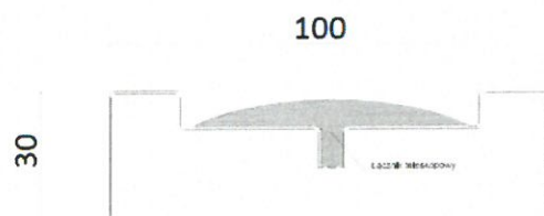
Rys. A2. Przekrój poprzeczny przekrycia dachowego DWW TYTANIUM PRUSZYŃSKI
