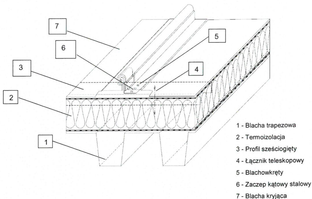
Rys. A1. Schemat przekrycia dachowego DWW TYTANIUM PRUSZYŃSKI
