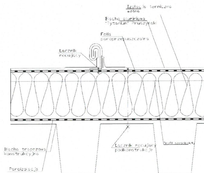
Rys. A2. Przekrój poprzeczny przekrycia dachowego DWW TYTANIUM PRUSZYŃSKI
