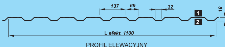
PROFIL ELEWACYJNY
