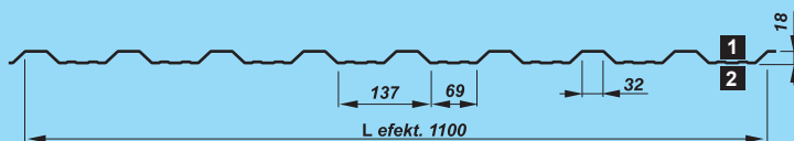
PROFIL DACHOWY
