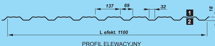
PROFIL ELEWACYJNY
