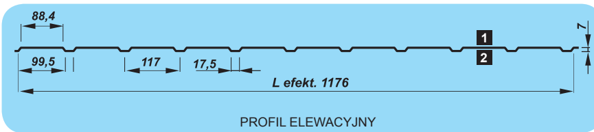
PROFIL ELEWACYJNY
