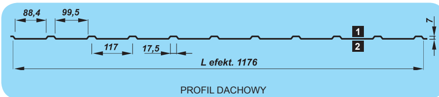
PROFIL DACHOWY
