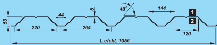
PROFIL ELEWACYJNY / KONSTRUKCYJNY
