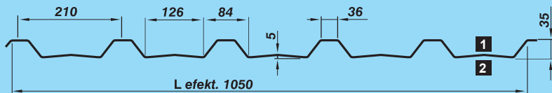
PROFIL DACHOWY
